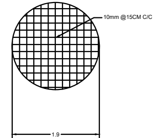
GRUND SLAB
